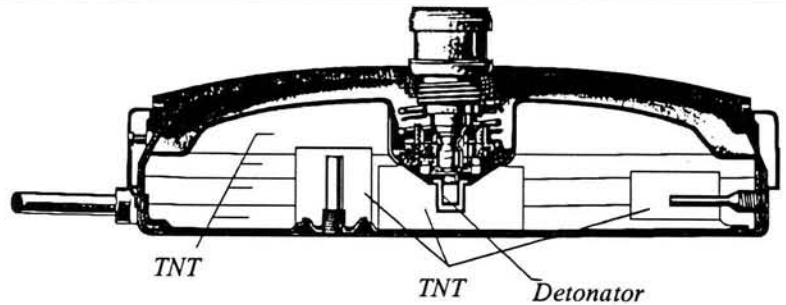
Die Duitse Tellermyn - sterk genoeg om die rusper van enige tenk af te skiet.
