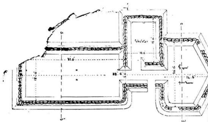
Fort Tullichewan se vloerplan.
